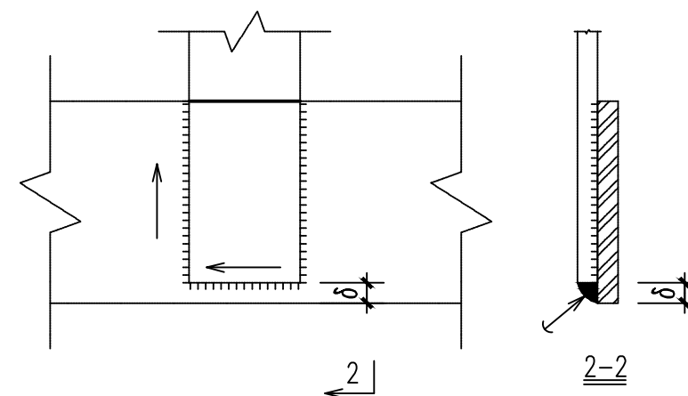
扁钢与扁钢垂直搭接详图
